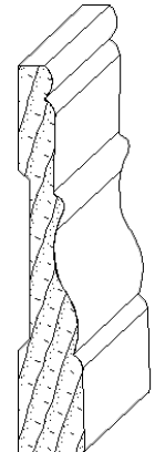
IH-4016 (178-A) 9/16 x 3-1/4 casing moulding
