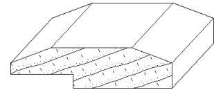
IH-804 1/2 x 2 flooring
